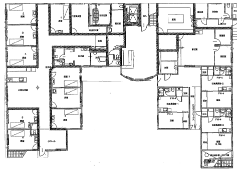
1F平面図
